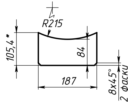
Поз.2 (Ребро)
