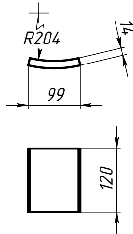
Поз.4 (Упор)
