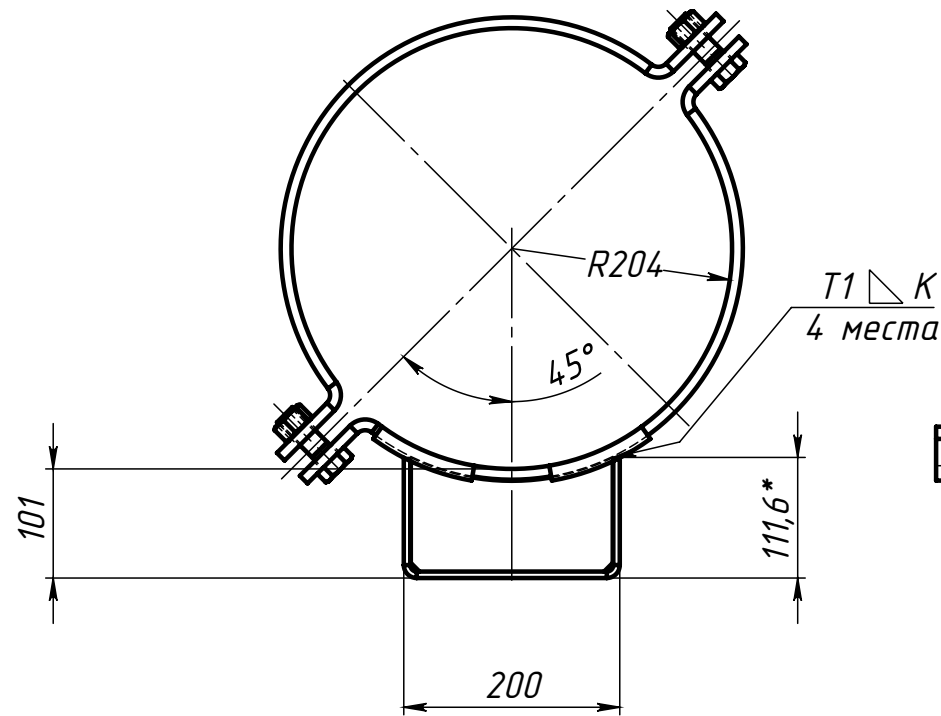
Поз.3 (Полухомут)
