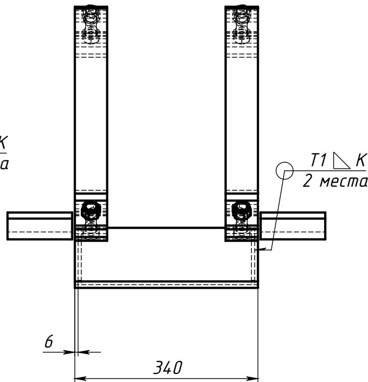
Поз.4 (Упор)
