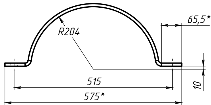
Поз.3 (Полухомут)
